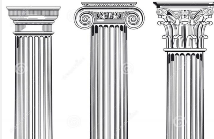
Columnas clásicas
