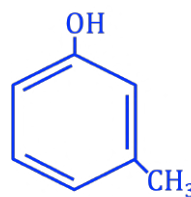
3-metilfenol m-cresol
