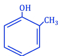
2-metilfenol o o-cresol
