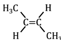
trans-2-buteno
