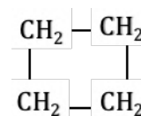
ciclobutano
