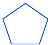
ciclopentano
