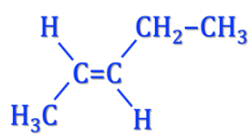
trans-2-penteno
