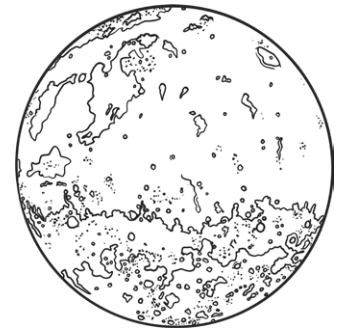
Mars
